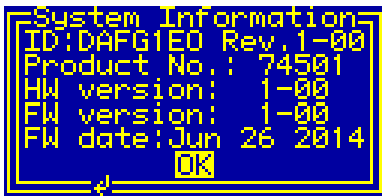
Fig. 53. Dialog box "System Information".
